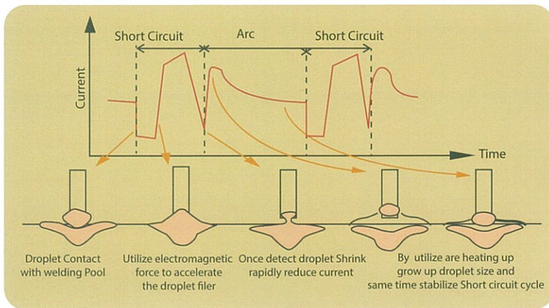
■ Workpiece Material : sus304(6mmt) ■ Wire size : \phi 1.2 ■ Current : 180A ■ Gas : 98%Ar+2% CO 2 ■ Voltage : 23V
